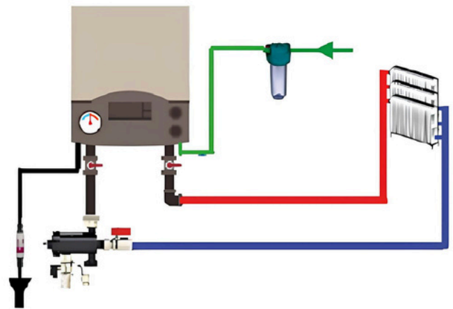
Installation de chauffage type
